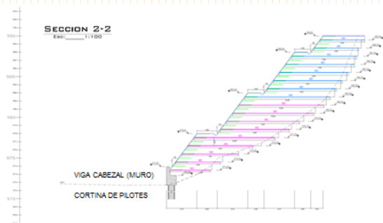
SECCION TRANSVERSAL DEL ÁREA AFECTADA SOLUCIÓN DE ESTABILIZACIÓN DEL TALUD (SIERRA®)
